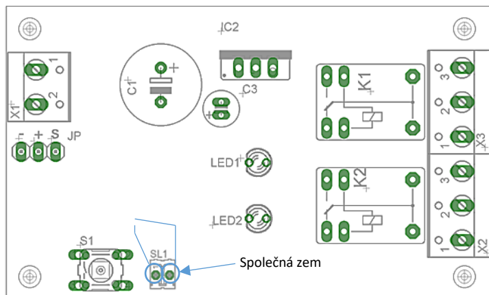
Rozložení konektorů na desce SVR v1.2
